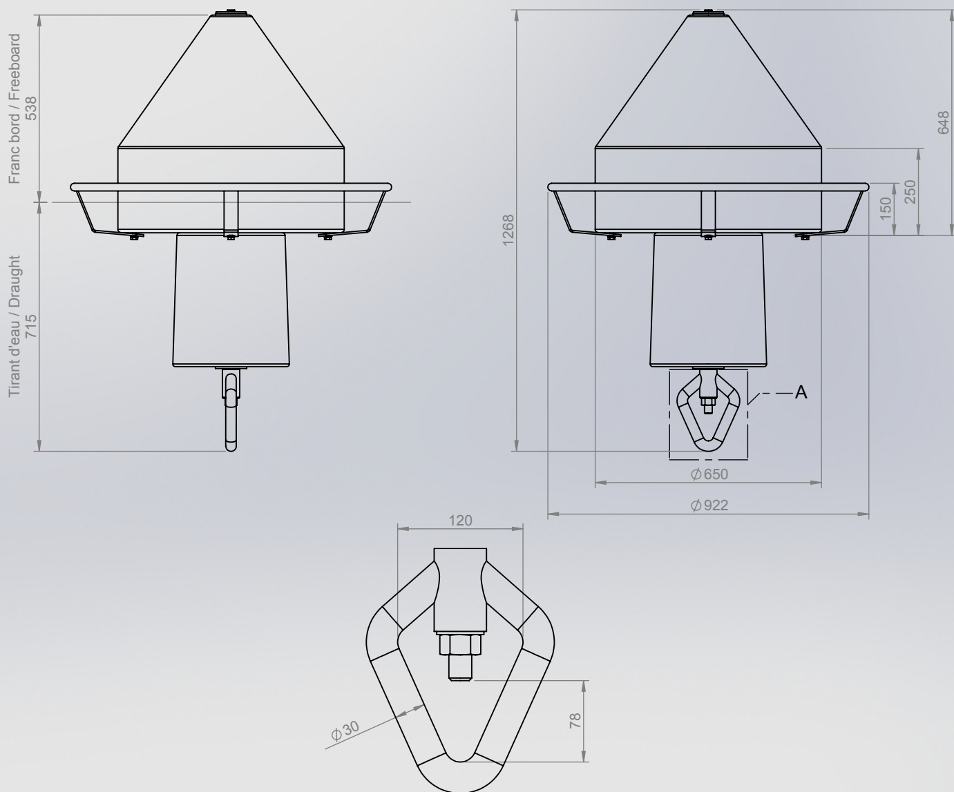
DÉTAIL A ECHELLE 1 : 5
